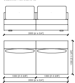
ELEMENTO SENZA BRACCIOILI / ELEMENT WITHOUT ARMS_200X105 2 SEDUTE DA 100 / 2 SEATS 100
