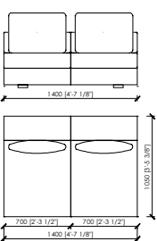
ELEMENTO SENZA BRACCIOILI / ELEMENT WITHOUT ARMS_140X105 2 SEDUTE DA 70 / 2 SEATS 70
