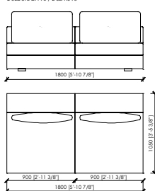
ELEMENTO SENZA BRACCIOILI / ELEMENT WITHOUT ARMS_180X105 2 SEDUTE DA 90 / 2 SEATS 90
