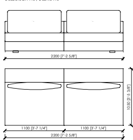
ELEMENTO SENZA BRACCIOILI / ELEMENT WITHOUT ARMS_220X105 2 SEDUTE DA 110 / 2 SEATS 110
